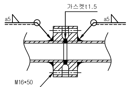
"C"부 상세도
