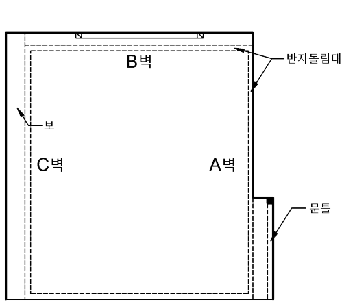
평면도
