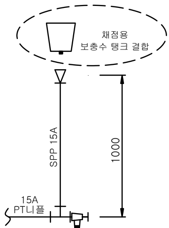
A - A' 상세도
