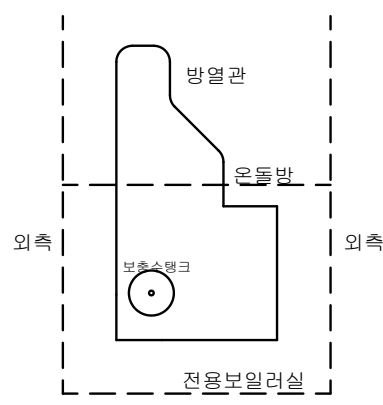
보일러 설치 배치도(평면도)
