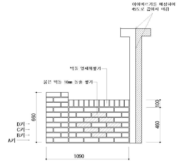
B방향 조적 쌓기
