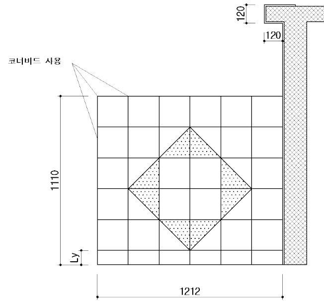
A-A' 방향 타일 붙임
