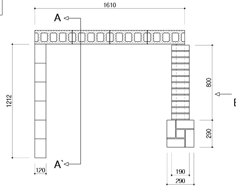
평면도
