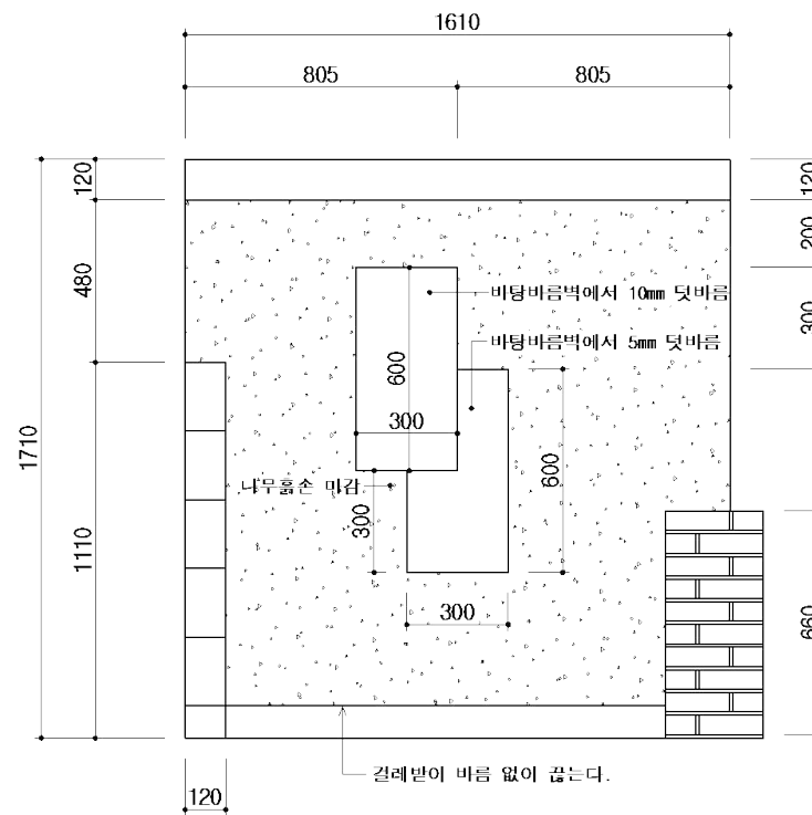
정면도
